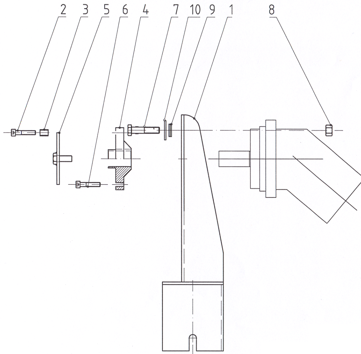
Antriebseinheit Hydraulisch Drive unit hydraulically CSA-1001 Pos. M
