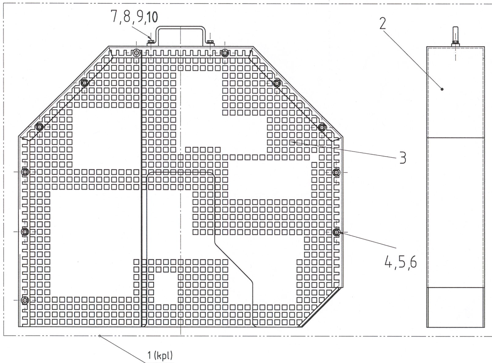
Antriebseinheit Radschutz Drive unit wheel protection CSA-1001 Pos. R
