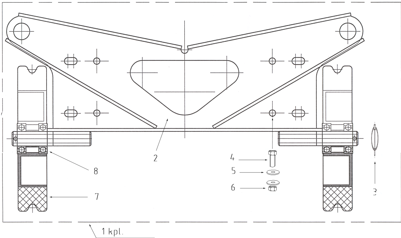
Fuss mit Räder Foot with wheels CSA-1001 Pos. B
