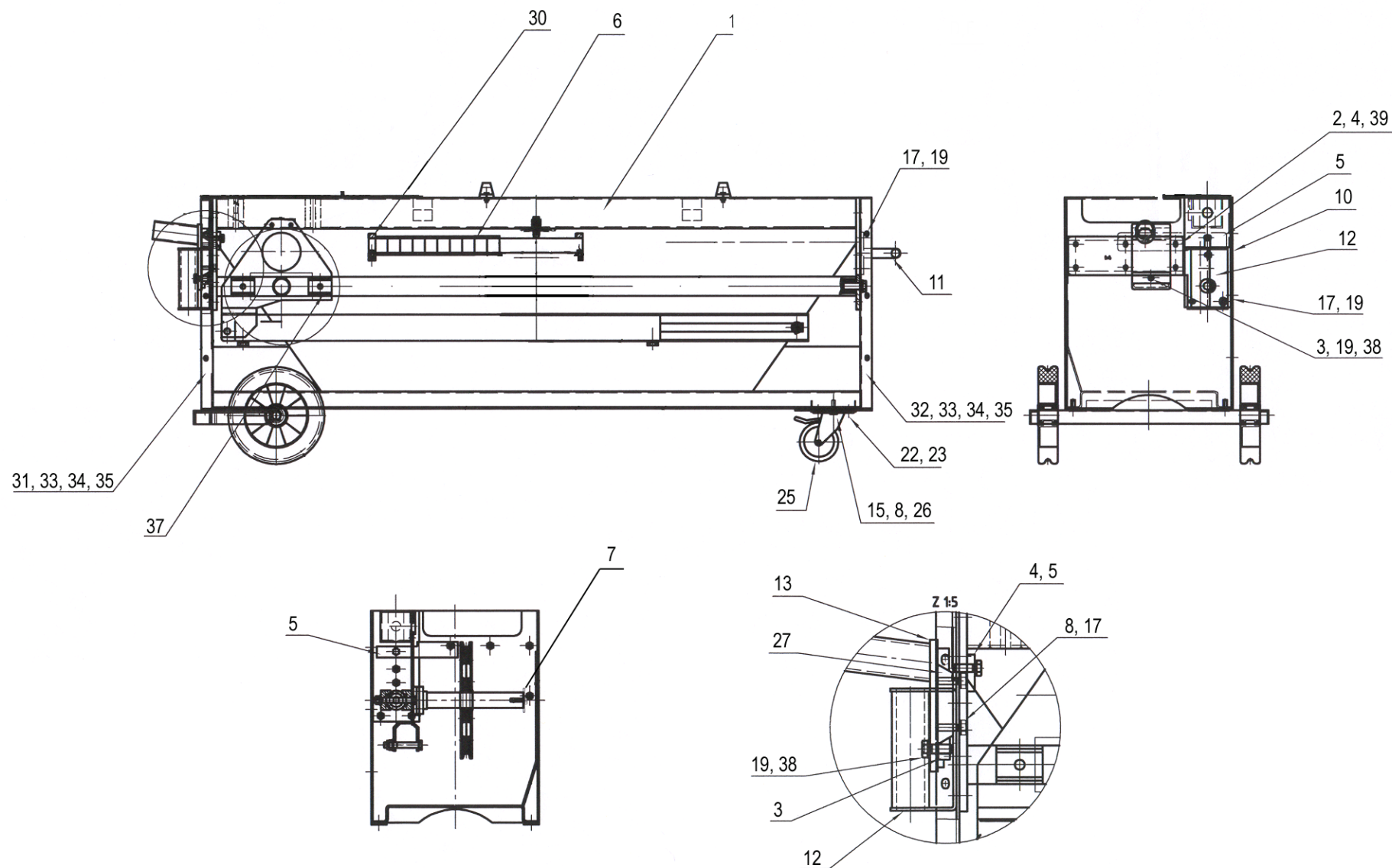
Innenrahmen Interiorframe CSA-1001 Pos. S
